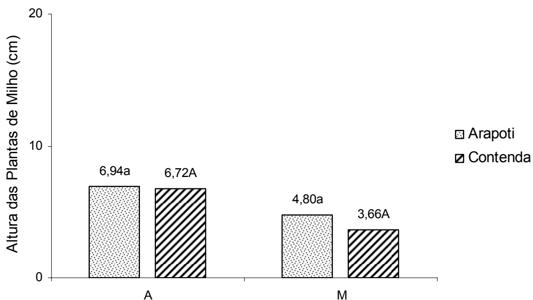
GRÁFICO 53 – ALTURA TOTAL DAS PLANTAS DE MILHO (EM cm) CULTIVADAS NO SOLO DE ARAPOTI E CONTENDA, SOB O TRATAMENTO NO PADRÃO DE MISTURA “D”
