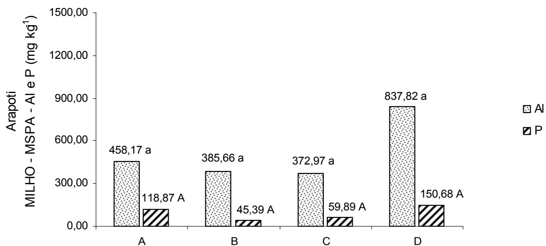
GRÁFICO 10 – TEORES TOTAIS DE Al E P ( \text{mg kg}^{-1} ) NAS PLANTAS DE MILHO CULTIVADAS NO SOLO DE ARAPOTI, SOB OS DIFERENTES TRATAMENTOS NO PADRÃO DE MISTURA “A”
