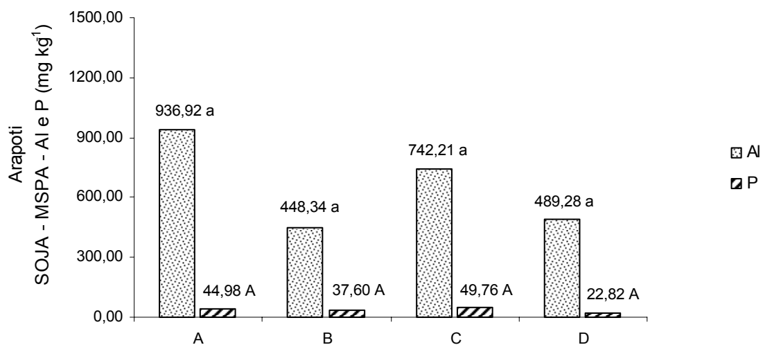
GRÁFICO 9 – TEORES TOTAIS DE Al E P ( \text{mg kg}^{-1} ) NAS PLANTAS DE SOJA CULTIVADAS NO SOLO DE ARAPOTI, SOB OS DIFERENTES TRATAMENTOS NO PADRÃO DE MISTURA “A”
