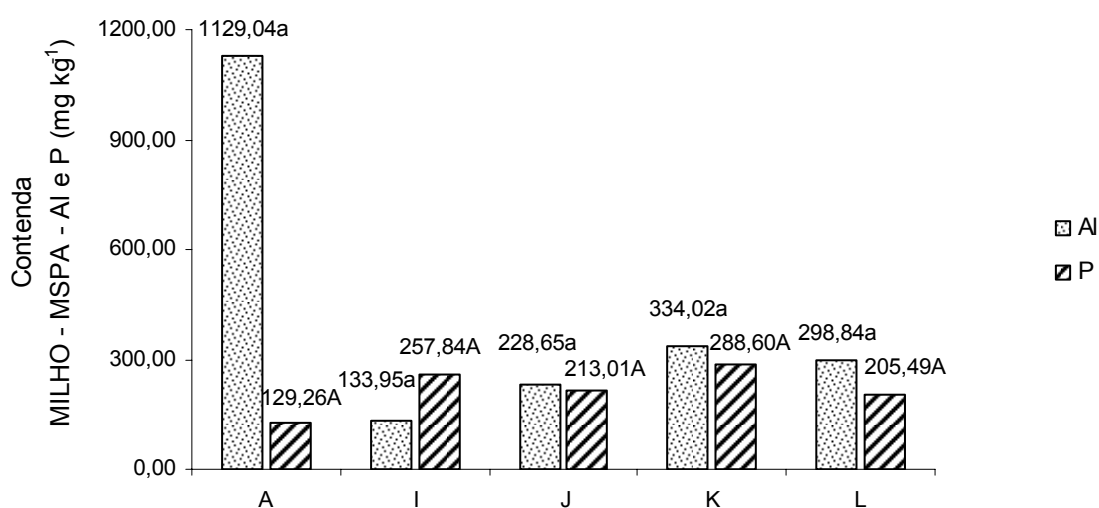
GRÁFICO 44 – TEORES TOTAIS DE Al E P (mg kg -1 ) NAS PLANTAS DE MILHO CULTIVADOS NO SOLO DE CONTENDA, SOB OS DIFERENTES TRATAMENTOS NO PADRÃO DE MISTURA “C”
